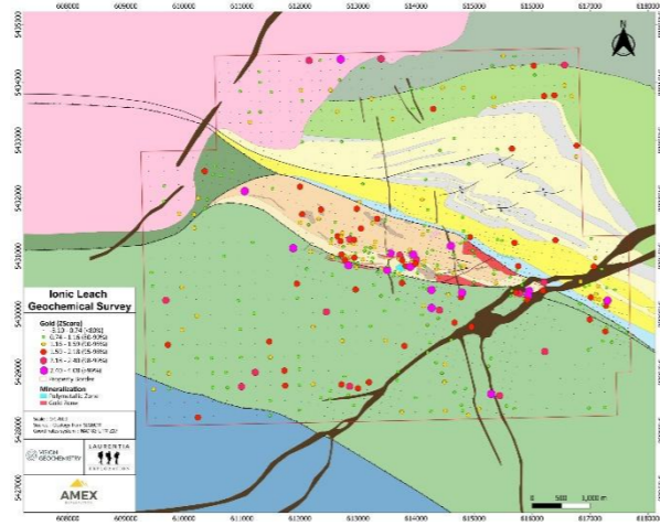
Au - Soil
