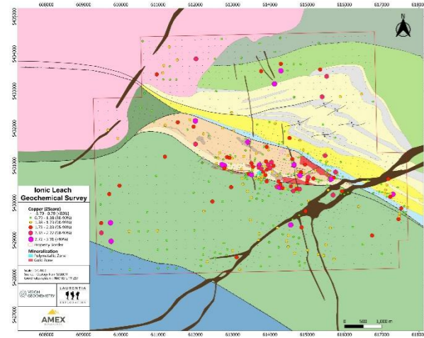
Cu - Soil
